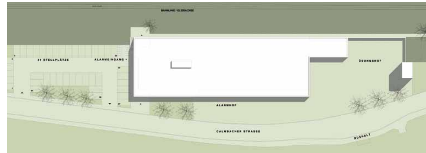
Lageplan des Feuerwehrhauses in Bad Wildbad
